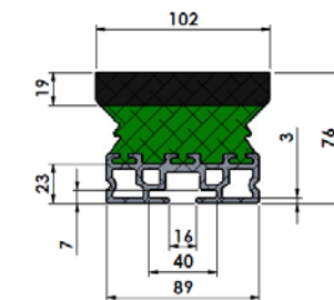
77 x 102 x 1400mm Load Zone Impact Bar V2
